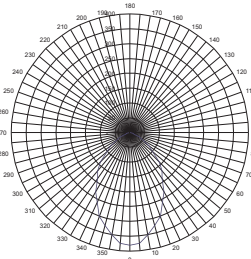
РСП-16-400-103
