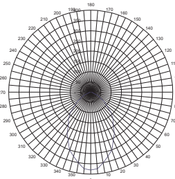
РСП-20-400-102
