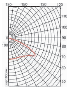
ЖКУ-13-150
