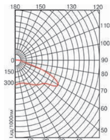
ЖКУ-13-100
