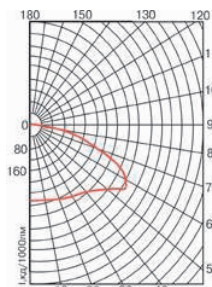
РКУ-13-125
